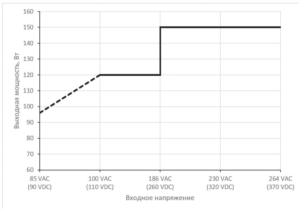
Рисунок А.7 - График зависимости максимальной выходной мощности от значения входного напряжения для КАН-Д120
