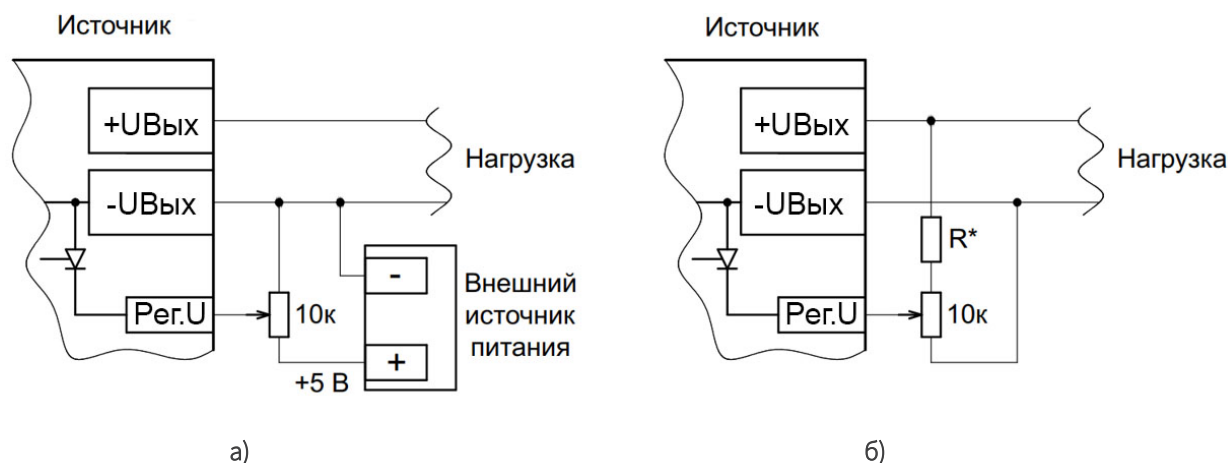
Рисунок 13 – Регулировка выходного напряжения с помощью вывода «Per.U» при подключении: а) к внешнему источнику питания +5 В; б) к выходу Источника.
